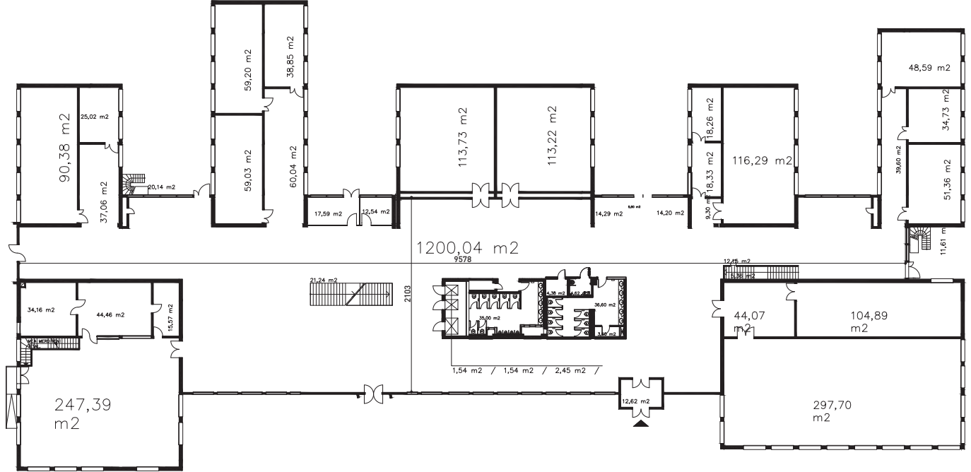
İLETİŞİM BİLİMLERİ FAKÜLTESİ EĞİTİM BLOĞU ZEMİN KAT PLANI
