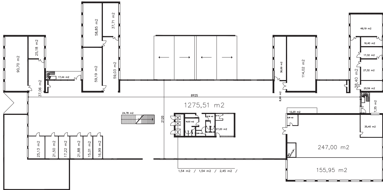
İLETİŞİM BİLİMLERİ FAKÜLTESİ EĞİTİM BLOĞU 3.KAT PLANI
