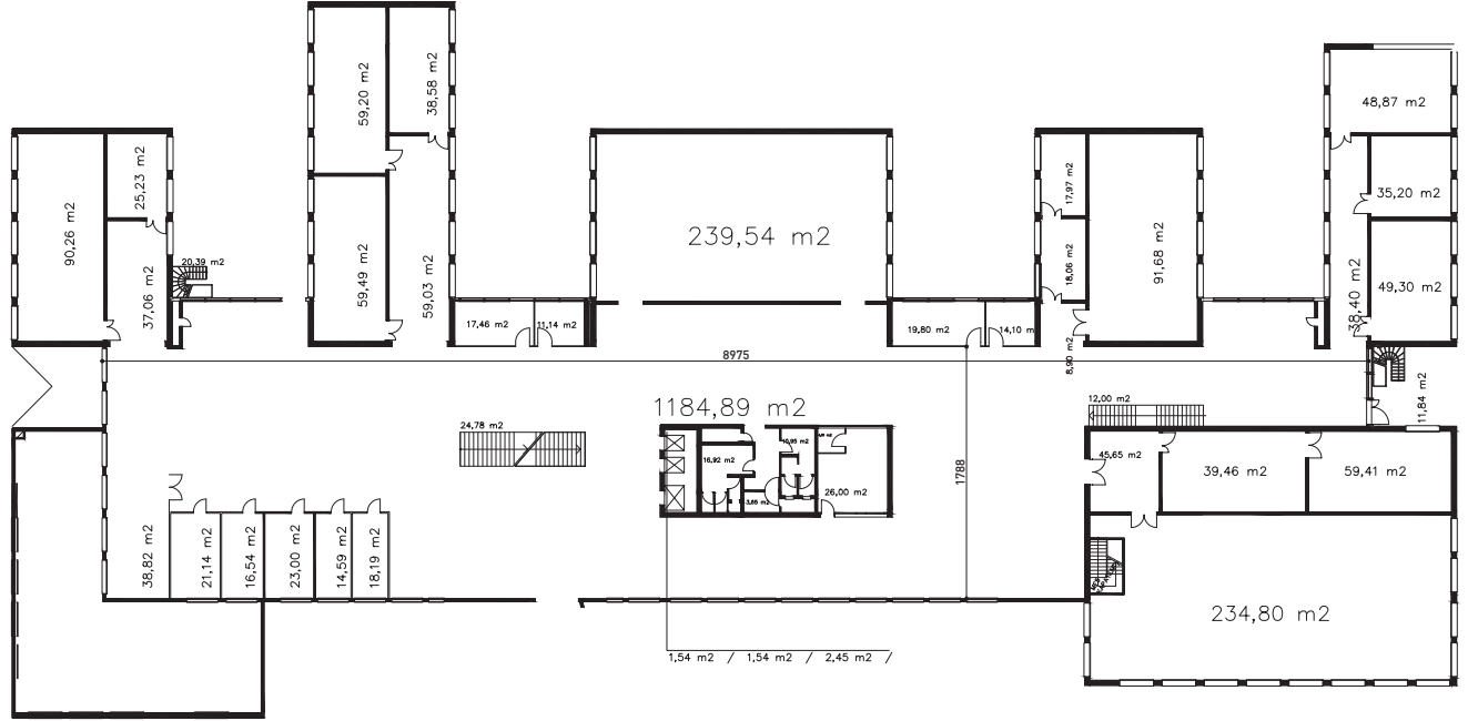
İLETİŞİM BİLİMLERİ FAKÜLTESİ EĞİTİM BLOĞU 2.KAT PLANI
